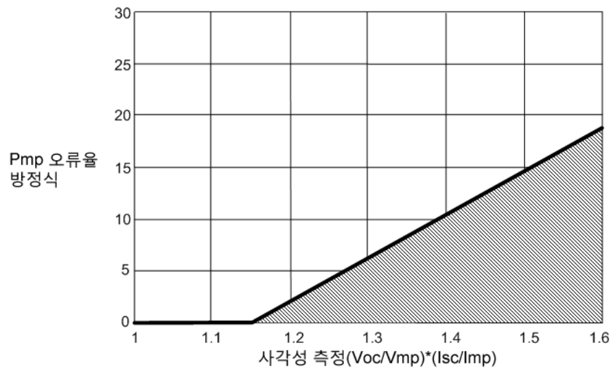
그림 A. 모델링 방정식으로 인한 Pmp 오류 범위
