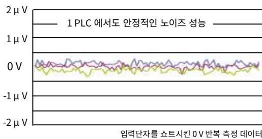
교정용 표준기에 다가서는 노이즈 성능 달성
