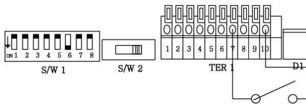
< 그림. 4-8 점점 스위치 입력방식 >
