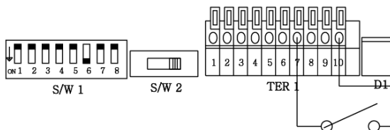
< 그림. 4-8 점점 스위치 입력방식 >
