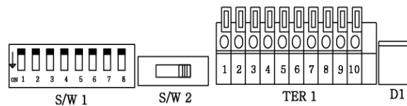
<그림. 4-2 Analog Control Terminal >
