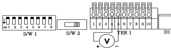
< 그림. 4-6 Remote Current Monitoring >
