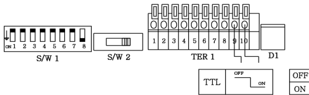
< 그림. 4-10 TTL Negative 입력방식 >
