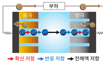
방전 중인 배터리 모식도
