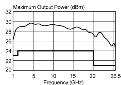
83018A Amplifier
