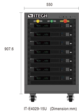
IT-E4029-15U (Dimension:mm)
